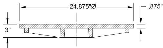
SECTION A-A
